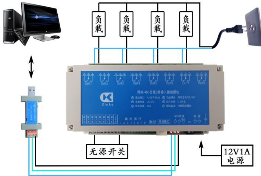
接线图示二（485总线控制）
